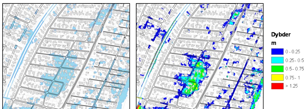
Figur 4.4 Udpegning af lavninger og beregninger af dybder.
