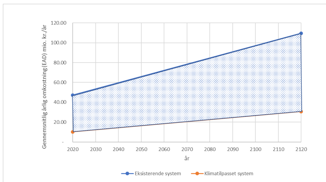
Figur 6.12 Illustration af beregning af skadesreduktion = skraveringen viser gevinsten i form af undgåede oversvømmelsesskader.
