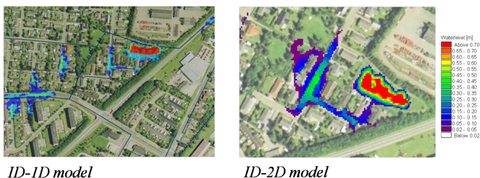
Figur 4.25 Resultater fra modeller med henholdsvis 1D og 2D overfladebeskrivelser.
