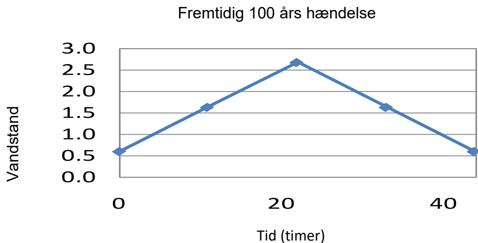
Figur 5.6 Eksempel på en tidsvarierende vandstand i havet – som input til en oversvømmelsesberegning.
