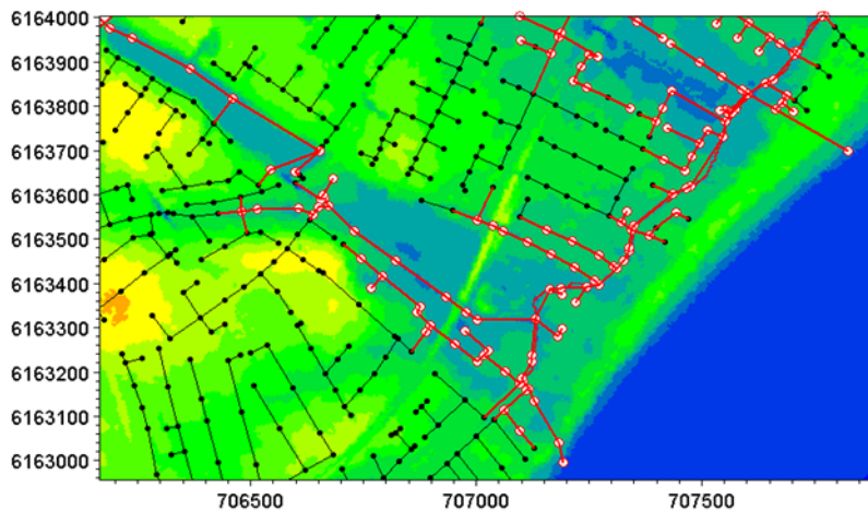
Figur 5.9 Kun udvalgte områder af afløbsmodellen (vist med rødt) er koblet til 2D strømningsmodellen. Dette sker for at optimere beregningstiden.
